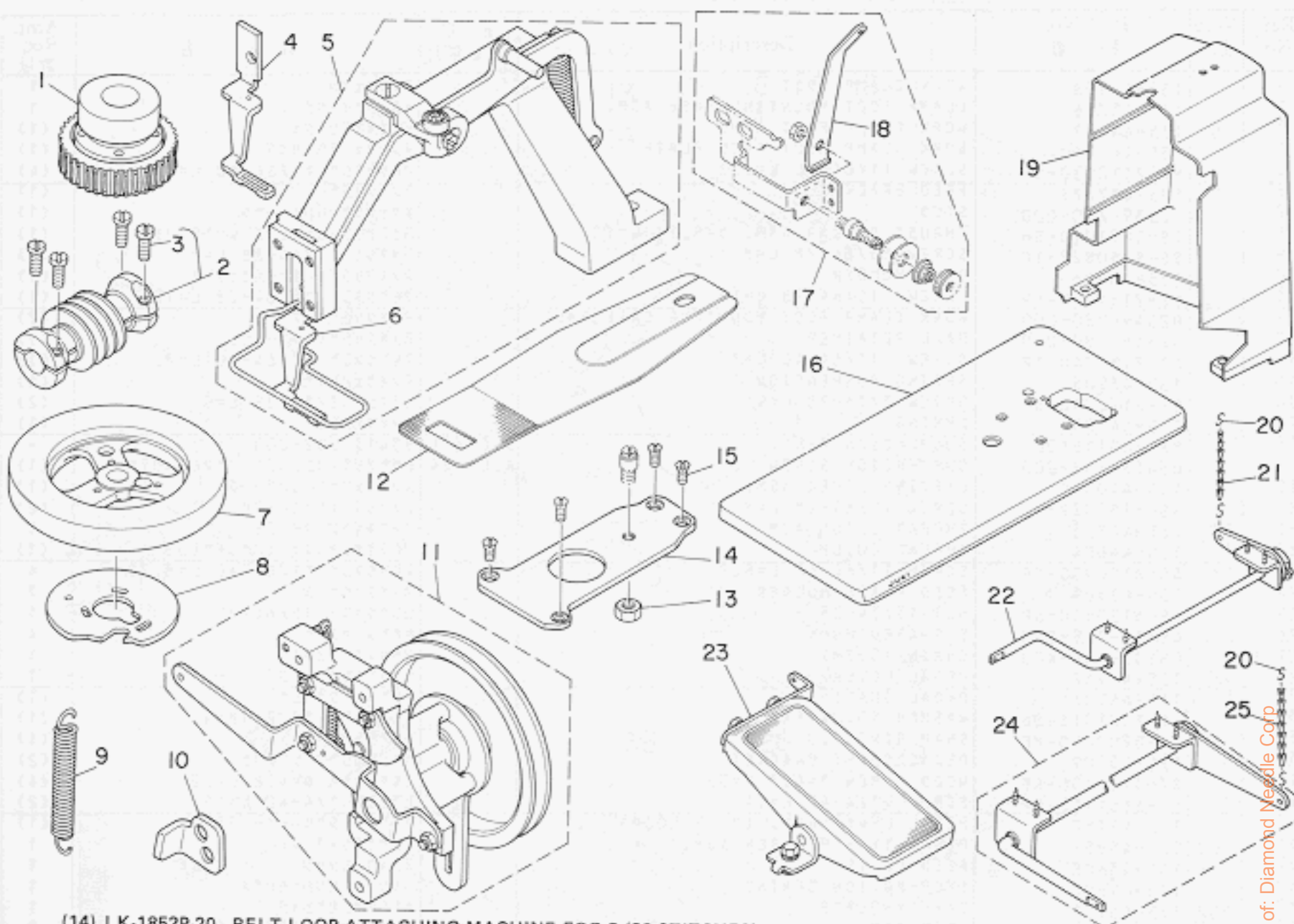
(14) LK-1852P-20 BELT LOOP ATTACHING MACHINE FOR P (28 STITCHES) P用28針バンドループ付けマシン
