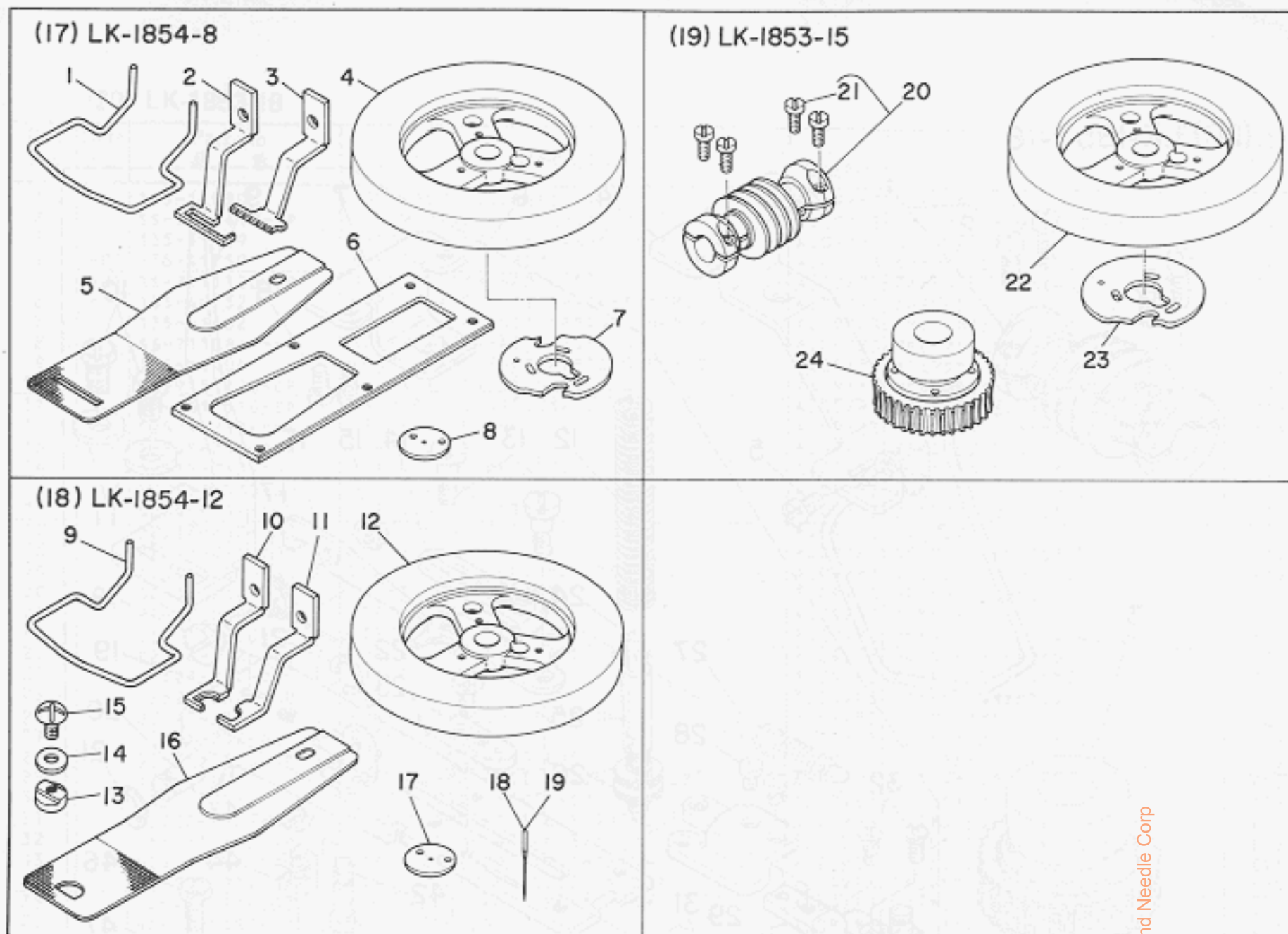
(17) LK-1854-8 LABEL TACKING MACHINE (21 STITCHES) ラベル付けマシン(21針)
