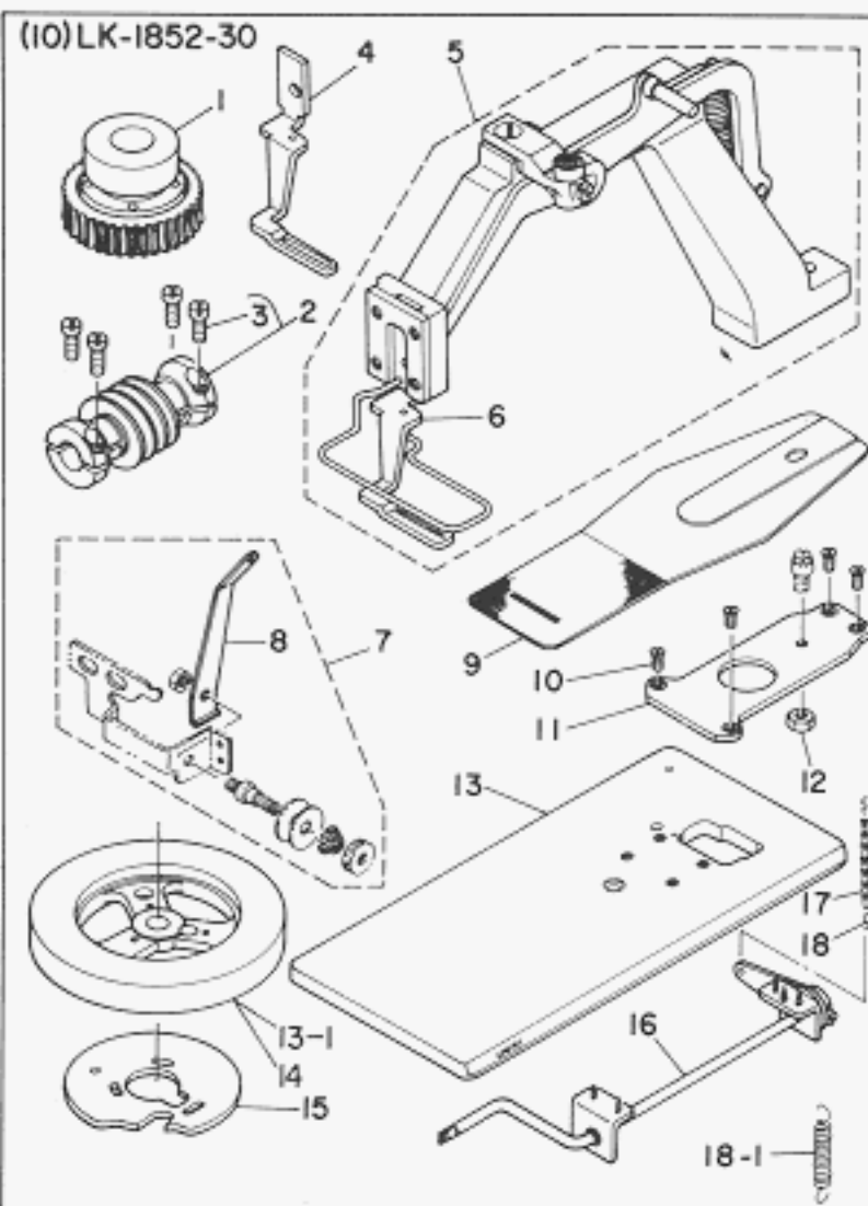
(10) LK-1852-30 BELT LOOP ATTACHING MACHINE (28 STITCHES) 28針バンドループ付けマシン
